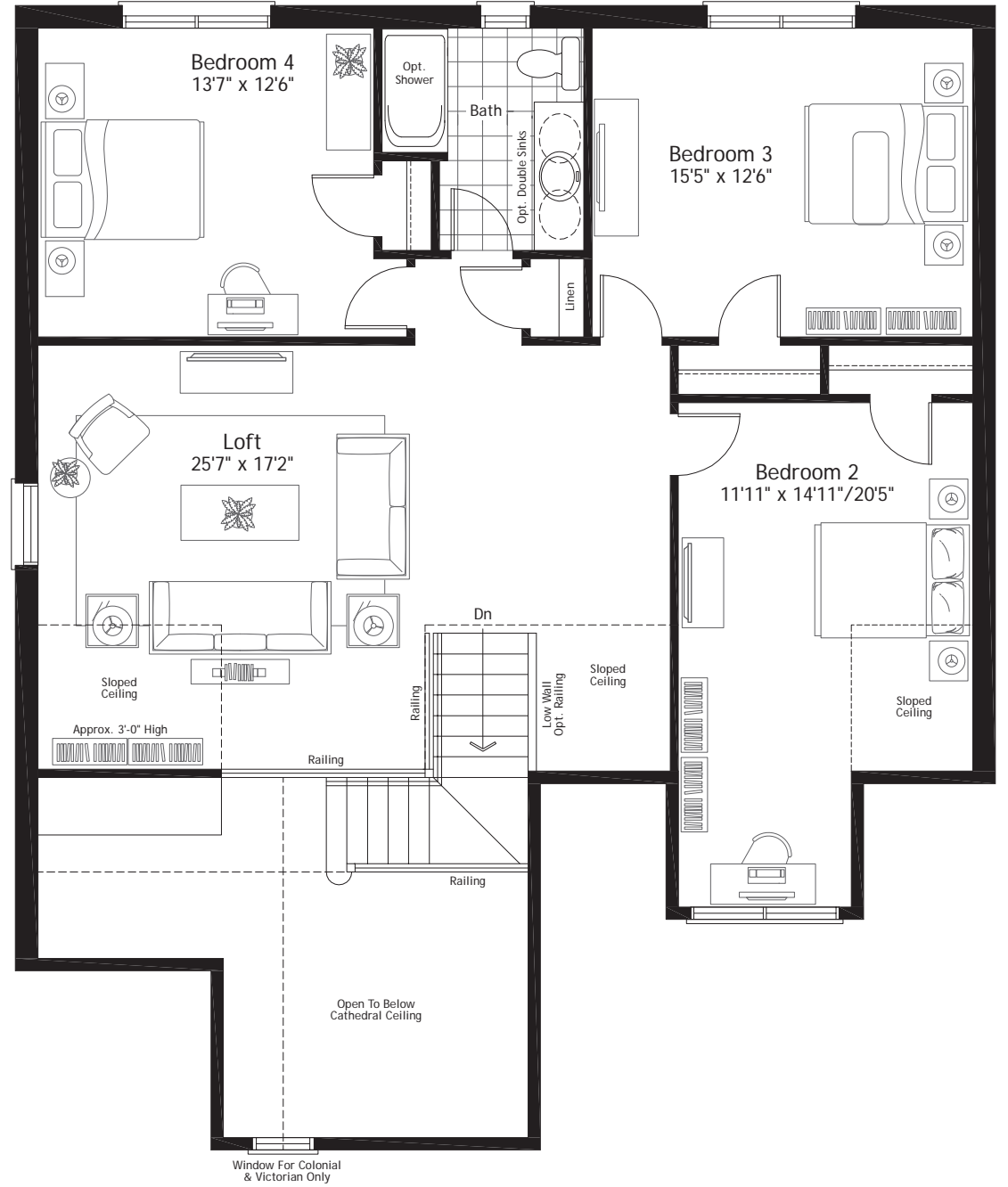
Loft Plan
